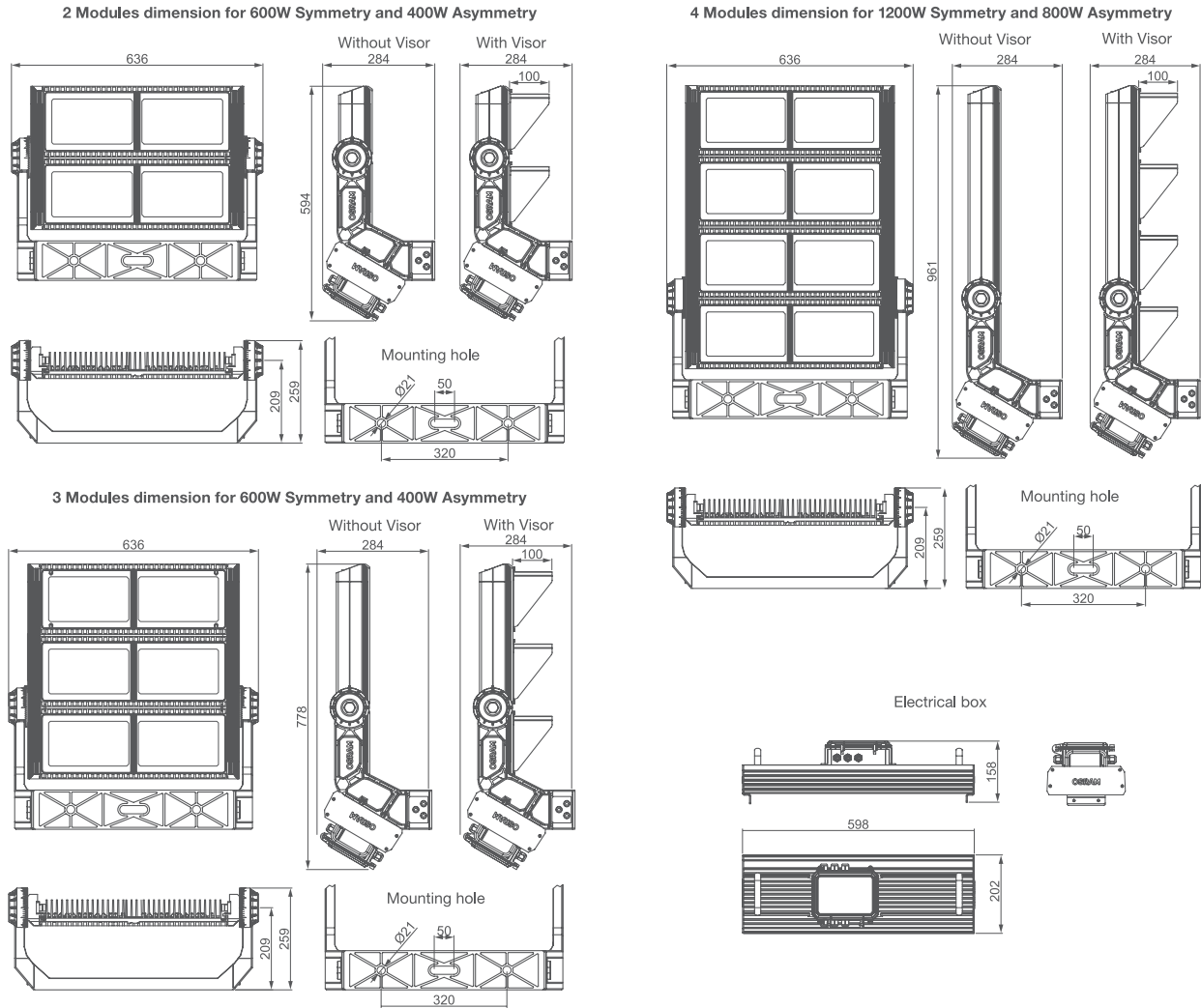
尺寸图
